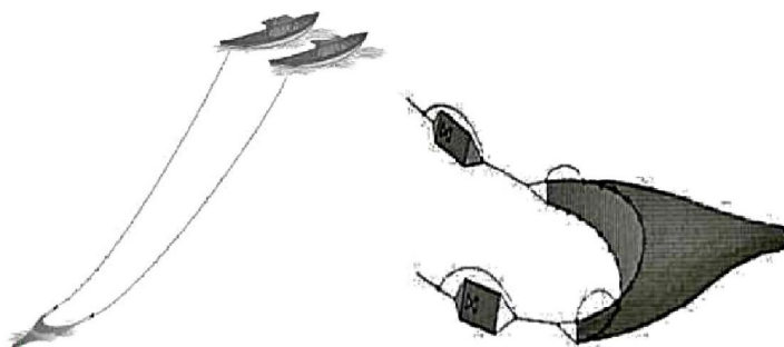
03.1.3 Pukat hela dasar dua kapal
